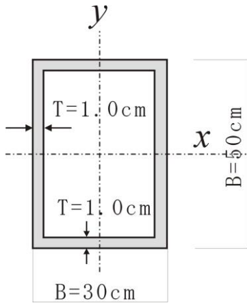
図 1 梁断面図
