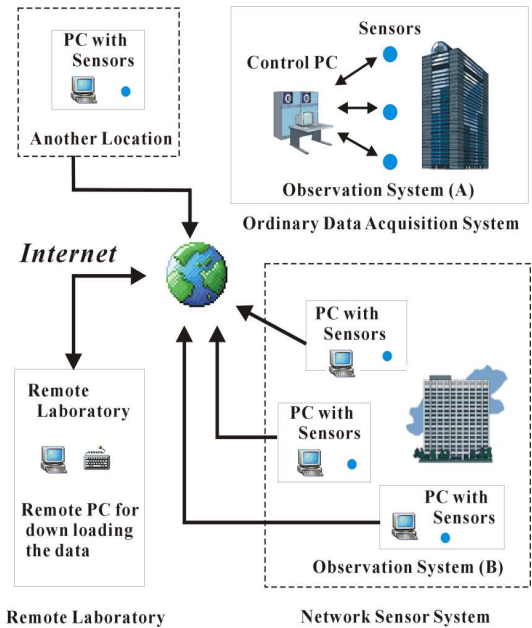
地震観測システム概要 (西村研究室)
